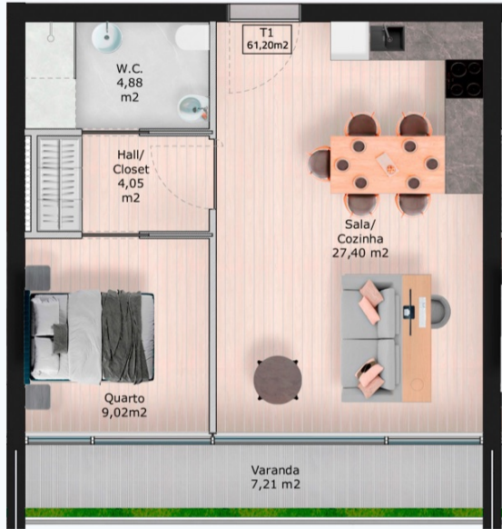
PISO 4: FRAÇÃO 4.5 TIPOLOGIA T1
