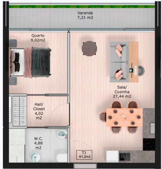
PISO 6: FRAÇÃO 6.1 TIPOLOGIA T1
