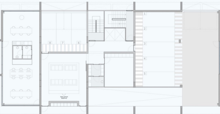
Piso Rês-do-chão
