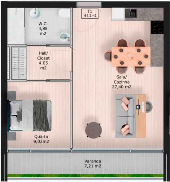
PISO 5: FRAÇÃO 6.4 TIPOLOGIA T1
