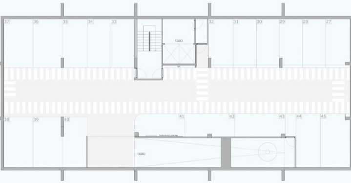
Piso -2
